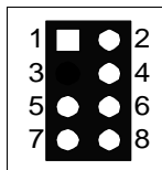
Bild 2-5: Pfostenstecker CN2
